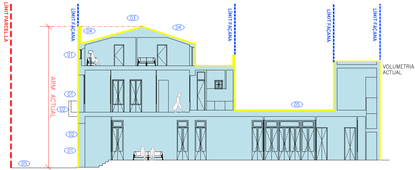
SECCIÓ LONGITUDINAL
