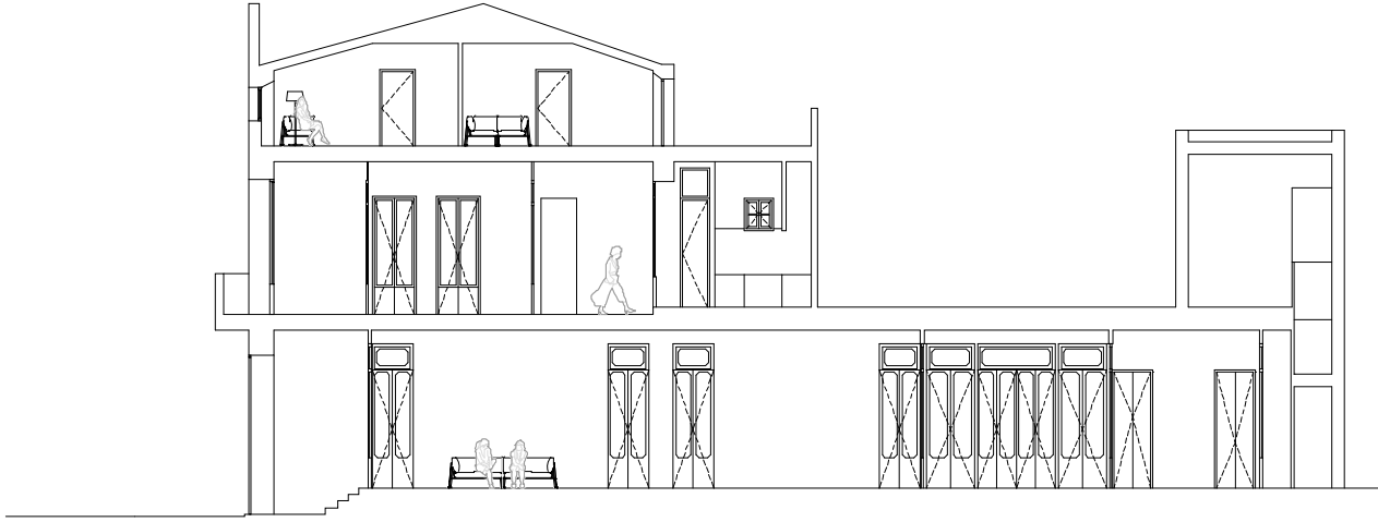
SECCIÓ LONGITUDINAL
