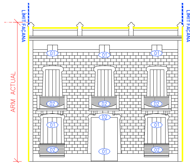
ALÇAT FAÇANA PRINCIPAL
