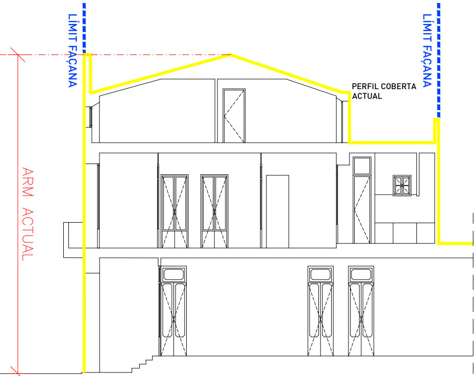
SECCIÓ LONGITUDINAL
